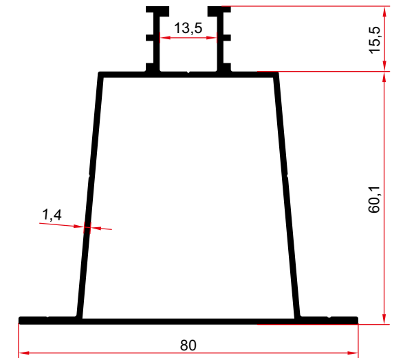
1361 1,171 Kg/m
