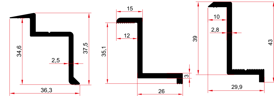
8028 0,456 Kg/m 2269 0,602 Kg/m 1102 0,528 Kg/m
