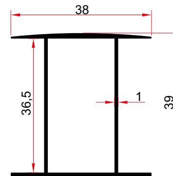
4778 0,421 Kg/m
