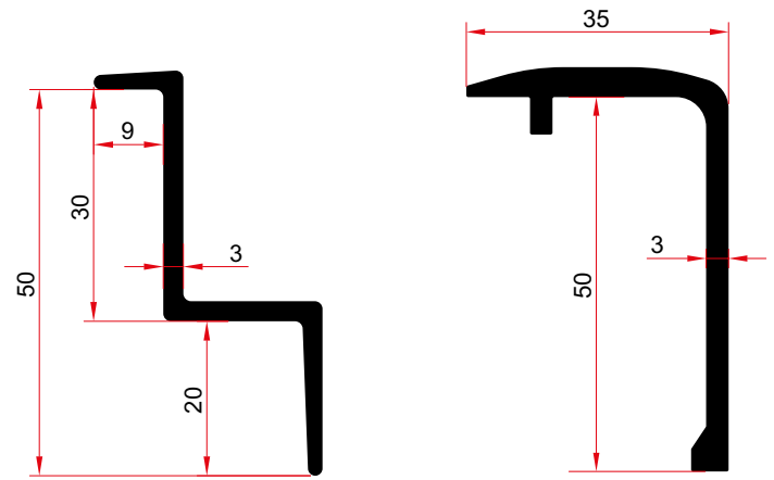
6103 0,526 Kg/m 6104 0,791 Kg/m
