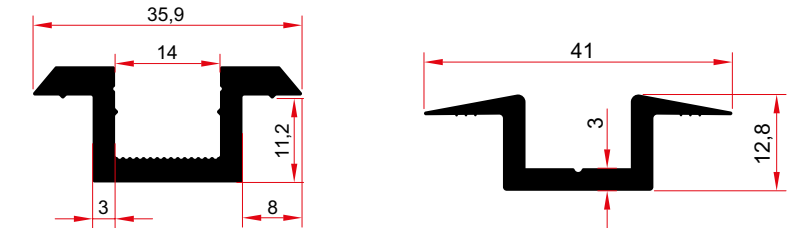
1329 0,518 Kg/m 1023 0,398 Kg/m
