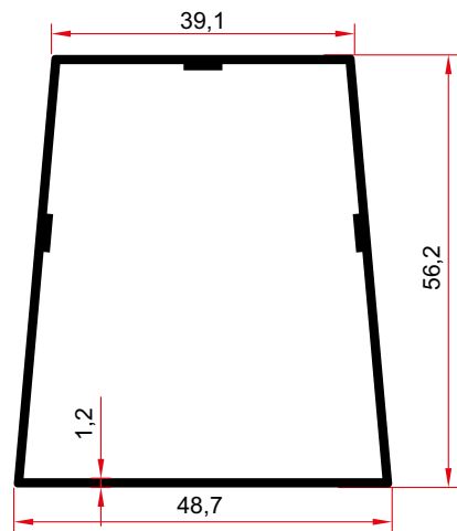
1021 0,669 Kg/m
