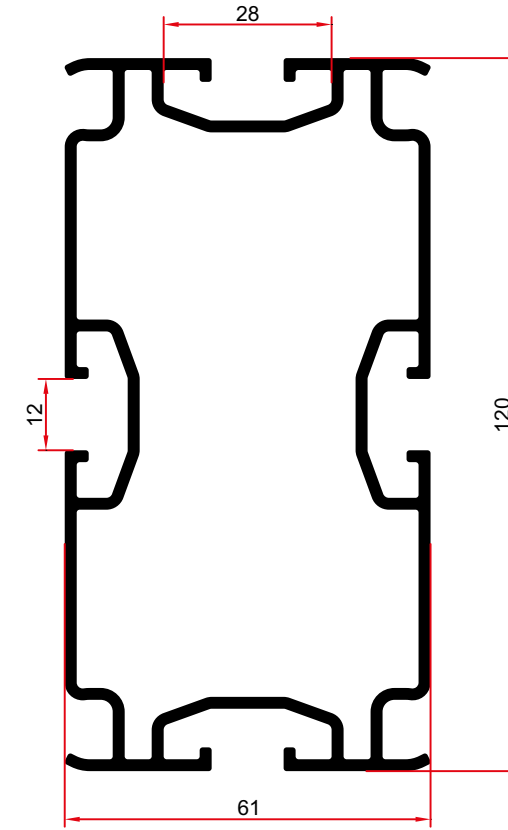
6105 2,808 Kg/m
