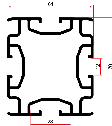
6100 2,266 Kg/m
