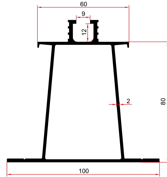
8035 2,030 Kg/m
