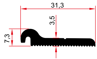
1022 0,314 Kg/m
