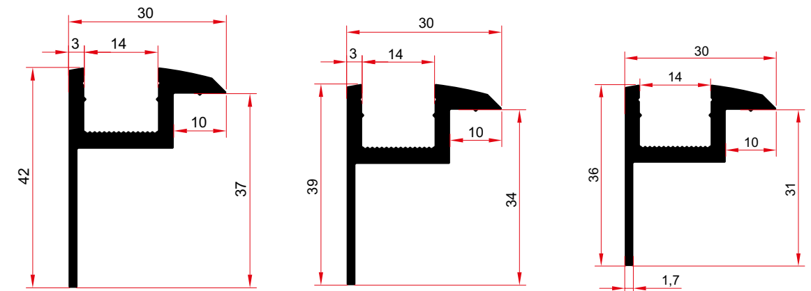
1331 0,585 Kg/m 1330 0,572 Kg/m 1608 0,558 Kg/m
