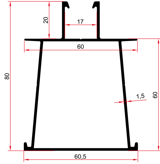
1020 1,130 Kg/m
